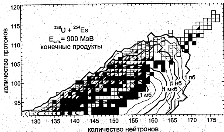
Рис. 7: Сечения образования конечных продуктов в реакции ^{238}\text{U} + ^{254}\text{Es} при E_{c.m.} = 900 МэВ, изображённые поверх карты известных нуклидов. Контурные линии показывают величину сечения в логарифмическом масштабе с шагом в один порядок.
