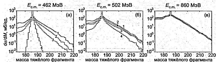
Рис. 4: Массовые распределения первичных продуктов реакции ^{160}\text{Gd} + ^{186}\text{W} , рассчитанные для трёх энергий E_{\text{c.m.}} = 462, 502 и 860 МэВ. Гистограммами показаны результаты для столкновений «вершина к вершине» (1), «вершина к боку» (2), «бок к вершине» (3) и «бок к боку» (4).
