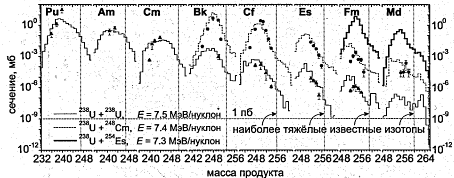
Рис. 6: Изотопные распределения конечных продуктов тяжелее мишени, полученные в столкновениях актинидов. Тонкие, пунктирные и толстые гистограммы соответствуют результатам расчётов для реакций ^{238}\text{U} + ^{238}\text{U} ( E = 7.5 МэВ/нуклон), ^{238}\text{U} + ^{248}\text{Cm} ( E = 7.4 МэВ/нуклон) и ^{238}\text{U} + ^{254}\text{Es} ( E = 7.3 МэВ/нуклон). Экспериментальные данные для реакции ^{238}\text{U} + ^{238}\text{U} (треугольники) взяты из [21], а для ^{238}\text{U} + ^{248}\text{Cm} (круги) — из работы [22]. Наиболее тяжёлые известные изотопы данных химических элементов обозначены вертикальными пунктирными линиями.
