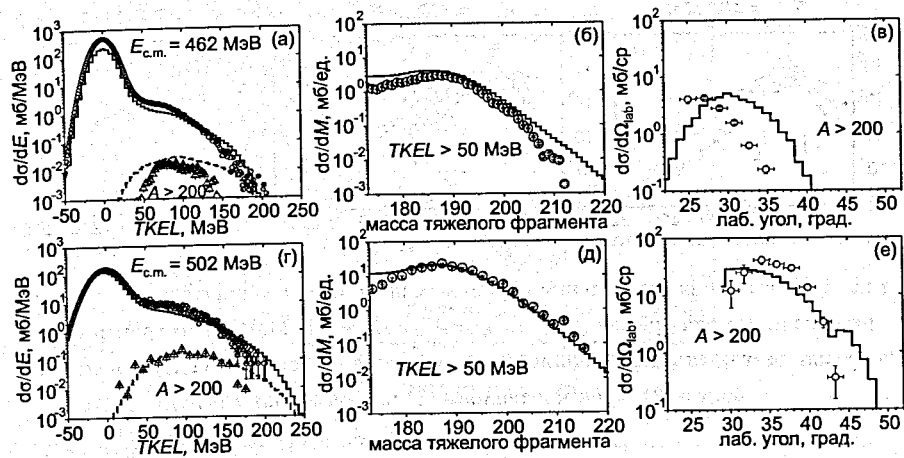
Рис. 5: Энергетические, массовые и угловые распределения первичных продуктов, полученных в реакции ^{160}\text{Gd} + ^{186}\text{W} при двух энергиях E_{\text{с.м.}} = 462 и 502 МэВ. Символами обозначены экспериментальные данные [12], жирные гистограммы показывают результаты расчётов, усреднённые по взаимным ориентациям ядер снаряда и мишени. Треугольниками и штриховыми гистограммами обозначены энергетические распределения, соответствующие мишенеподобным фрагментам с A > 200 . В расчётах учитывалось экспериментальное разрешение (FWHM) 12 МэВ по энергии и 3 единицы по массе.
