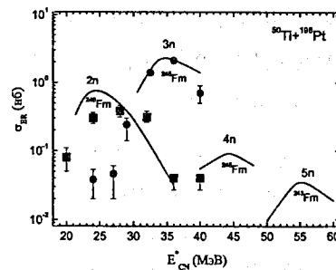
Рис.1. Рассчитанные (сплошные линии) сечения* Рис.2. То же, что и на рис.1, но для реакции функций возбуждения и испарительных остатков для указанных 2n испарительных каналов в реакции ^{50}\text{Ti} + ^{198}\text{Pt} . Экспериментальные данные показаны значками.
