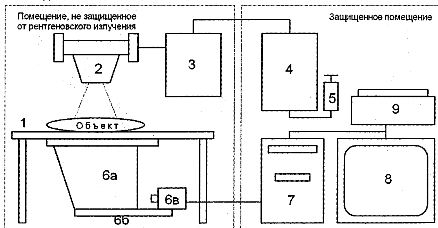
Состав и размещение приставки.
