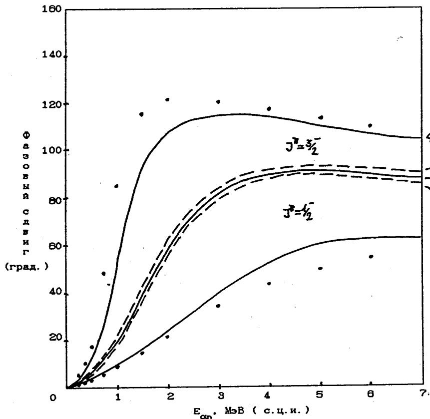
Фазы \alpha -рассеяния. Точки – эксперимент. 1 – «средняя» экспериментальная фаза. 2,3 – фазы, отвечающие реалистическим NN-силам с увеличенным притяжением, без учета спин-орбитальных сил. 4,5 – фазы, рассчитанные с учетом реалистических ls -сил.
