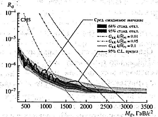
Рис. 8. Пределы на массу RS-гравитонов в комбинированном канале e^+e^- + \mu^+\mu^- [6, 11].
