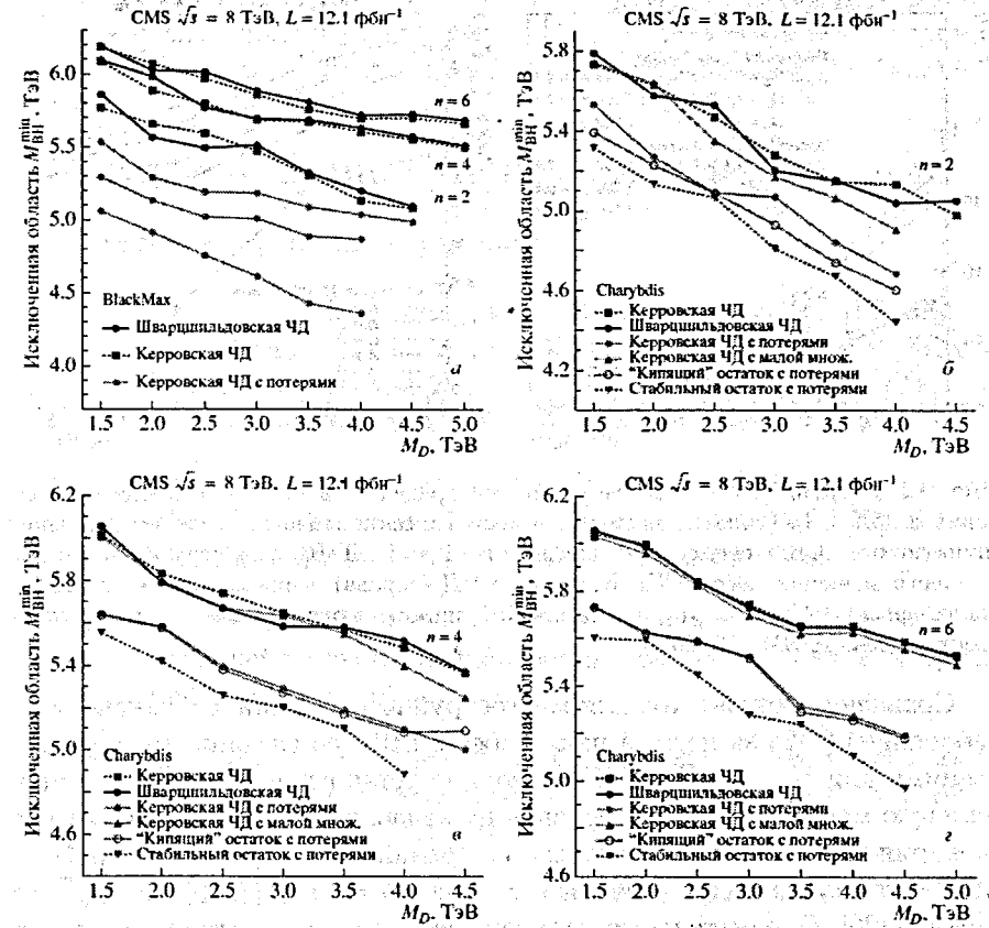
Рис. 11. Исключенная (95% C.L.) минимальная масса ЧД в зависимости от величины M_D для различных моделей ЧД в генераторах (а) BLACKMAX и (б) — (г) SNARYBDIS2. Области под кривыми считаются закрытыми [10, 11, 20].
