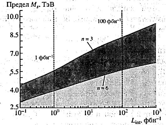
Рис. 3. Достижимый предел \sigma со статистической значимостью 5\sigma на значения M_S для числа дополнительных измерений n = 3, 4, 5, 6 [1, 12].
