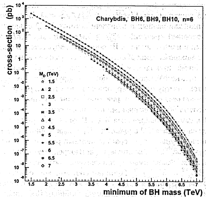
Рис. 9. Сечения рождения ЧД для \sqrt{s} = 8 ТэВ в зависимости от минимальной массы M_{BH}^{min} для различных значений M_D и числа дополнительных измерений n = 6 . Вычисление потерь проводилось по механизму Йошино–Рычкова [19].
