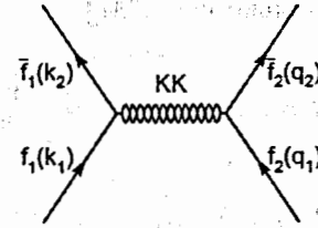
Рис. 1. Процесс четырехфермионного взаимодействия с обменом КК–модами гравитонов.
