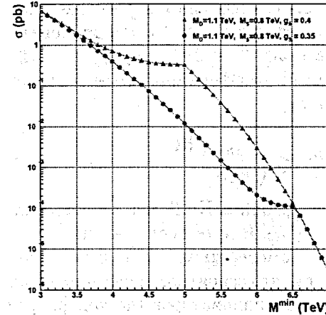
Рис. 10. Смена режимов СШ/ЧД и сшивка сечений для разных выборов g_S .
