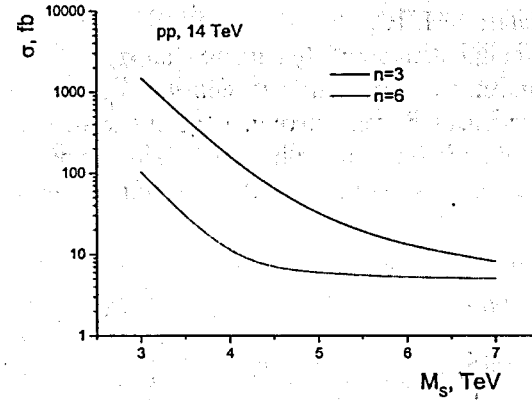
Рис. 2. Сечение рождения пары мюонов с M_{inv} \geq 1 ТэВ/с 2 при \sqrt{s} = 14 ТэВ с учетом вклада ADD-гравитонов в зависимости от M_S для двух крайних рассчитанных значений n = 3 (верхний) и 6 (нижний).
