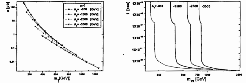
Рис. 5: Слева представлены сечения рождения пар топ-скварков как функции массы m_{\tilde{t}} . Справа показана зависимость времени жизни легчайшего топ-скварка от параметра m_{1/2} для различных значений A_0 .
