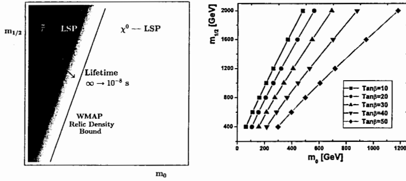
Рис. 2: Слева показана область коаннигиляции в плоскости (m_0 - m_{1/2}) . Справа показано как разрешенная область меняется с изменением \tan \beta . Значения \tan \beta растут слева направо.
