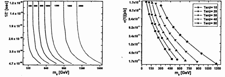
Рис. 3: Слева показано время жизни \tilde{\tau} в сек, как функция параметра m_0 вблизи границы для \tan \beta = 50 . Значения параметра m_{1/2} растут слева направо. Справа представлены сечения рождения для пары слептонов на ЛНС в пикобарнах, как функции параметра m_0 для различных значений \tan \beta в области коаннигиляции.
