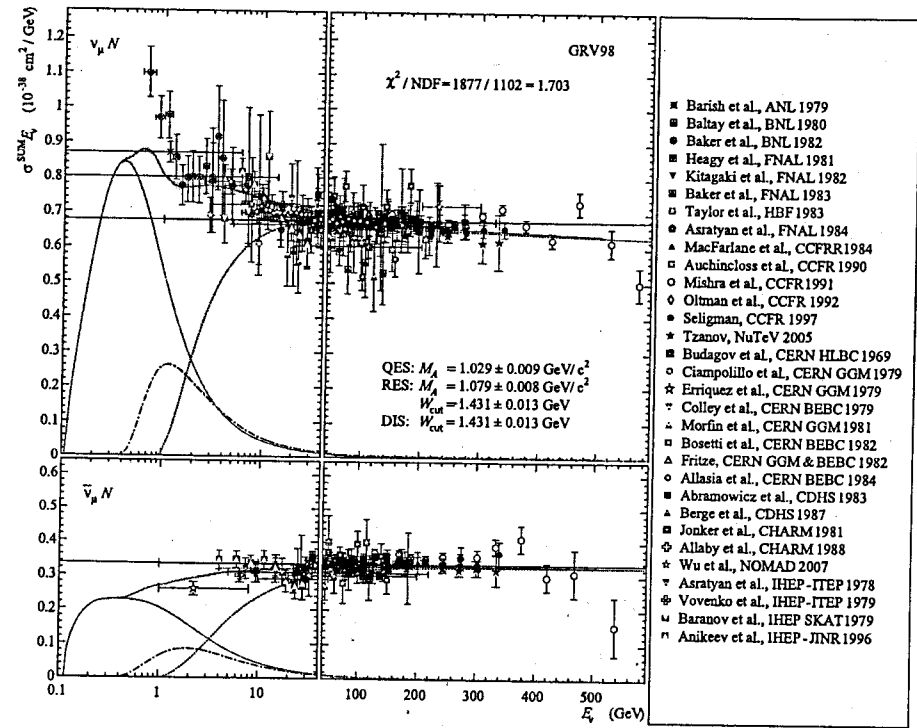
Рис. 2: Полные суммарные сечения реакций рассеяния \nu_\mu и \bar{\nu}_\mu на изоскалярных нуклонах, нормированные на энергию (анти)нейтрино, измеренные в экспериментах ANL, BNL, FNAL, CERN и IHEP. Данные, исключенные из глобального анализа, показаны бледными символами. Сплошными линиями показаны «мировые средние значения» для сечений реакции \nu_\mu N и \bar{\nu}_\mu N , полученные Particle Data Group [16]. Сечения квазиупругих реакций рассчитаны с использованием ВВВА(07) модели векторных форм-факторов нуклонов; сечения реакций одиночного резонансного рождения пионов рассчитаны с модифицированной моделью Рейна-Сегала, с учетом нерезонансного фона; структурные функции сечений глубоконеупругих реакций рассчитаны с моделью партонных распределений GRV98. В расчетах использованы значения параметров M_A^{\text{QES}} , M_A^{\text{RES}} , W_{\text{cut}}^{\text{RES}} и W_{\text{cut}}^{\text{DIS}} , полученные из глобального статистического анализа. Показаны сечения QES, RES и DIS вкладов и суммарные сечения (для сечений антинейтрино показана сумма сечений QES и QHP). Закрашенными полосами показаны неопределенности в сечениях, вызванные неопределенностями в значениях аксиальных масс и обрезаний.
