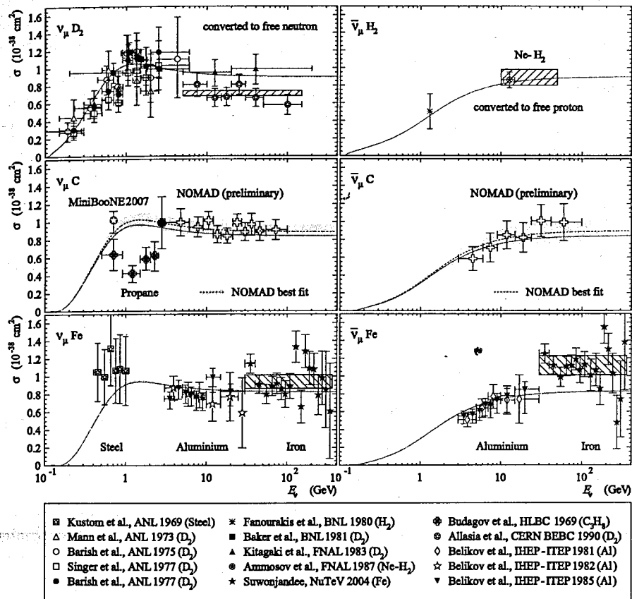
Рис. 1: Полные сечения квазиупругих реакций \nu_\mu n и \bar{\nu}_\mu p , измеренные в экспериментах с дейтериевыми, водородными, углеродными (пропановыми), алюминиевыми и железными (стальными) мишенями. Экспериментальные данные, исключенные из анализа, показаны бледными символами. Сплошными кривыми показаны сечения, рассчитанные с ВВВА(07) моделью векторных форм-факторов нуклонов, для значения M_A^{\text{QES}} = 0.999 \pm 0.011 \text{ ГэВ}/c^2 , полученного из совместного статистического анализа данных полных и дифференциальных сечений квазиупругих реакций \nu_\mu n и \bar{\nu}_\mu p . Пунктирными кривыми показаны сечения, вычисленные с GKex(05) моделью векторных форм-факторов нуклонов, для значений M_A^{\text{QES}} , полученных из анализа предварительных данных эксперимента NOMAD [5]. Закрашенными полосами показаны неопределенности в сечениях, вызванные неопределенностями в значениях M_A^{\text{QES}} .
