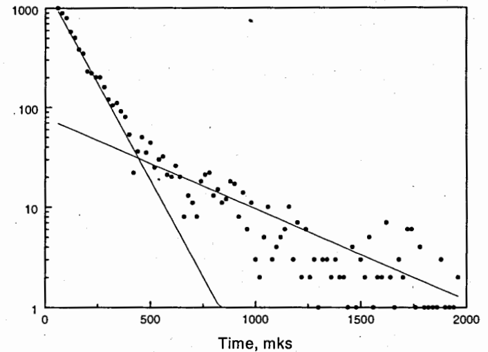
Рис. 1. Сигнал ИНК (счет нейтронов во временном окне 20 мкс). 1 - короткоживущая (скважинная) компонента, 2 - долгоживущая (пластовая) компонента
