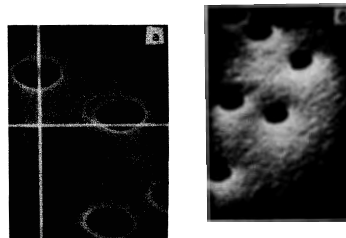
Рис. 1. Электронные микрофотографии ядерных мембран на основе ПП-пленок, облученных ионами ксенона с полной энергией 125 МэВ. Плотность пор 10^7 \text{ см}^{-2} : а/ мембрана на основе пленки I. Увеличение 9300. Вертикальная и горизонтальная
