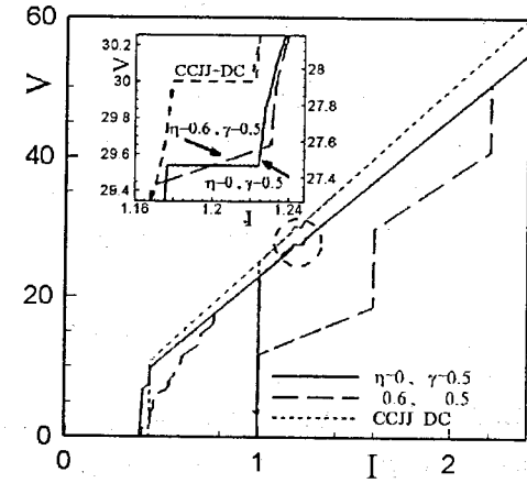
Рис. 8. ВАХ стека СДП без зарядового разбаланса \eta = 0 (сплошная линия) и с учетом разбаланса при \eta = 0.6 (линия крупным пунктиром). Для сравнения показаны результаты, полученные в рамках модели CCJJ + DC при перидических граничных условиях (линия мелким пунктиром). Увеличенная часть ВАХ со ступенькой Шапиро показаны на вставке.
