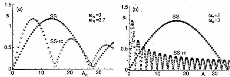
Рис. 3. (а) Амплитудная зависимость ширины ступеньки W на резонансной ветви (SS-rc) при \omega_R = 2.7 по сравнению с зависимостью без шунтирования (SS). Точки показывают численно рассчитанную амплитудную зависимость ширины ступеньки Шапиро без шунтирования (SS, синие точки) и с шунтированием (SS-rc, красные точки). Квадраты показывают аналитические результаты для случая без шунтирования (SS, синие квадраты) и результаты подгонки для шунтированного ДП (SS-rc, красные квадраты). (б) То же, что и на рис. 3(а) при \omega_R = 3 .
