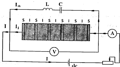
Рис. 1. Схема системы джозефсоновских переходов с LC-шунтированием
