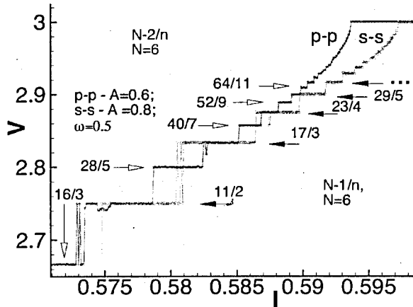
Рис. 6. (а) Лестничная структура ДП с p -спариванием (при A \approx 0.6 ) и s -спариванием (при A = 0.8 ) для параметра прозрачности D = 0.7 и \omega = 0.5 . Стрелками отмечены дополнительные последовательности характерные для ДП с p -спариванием. (б) То же, что и в (а), но с разными амплитудами внешнего излучения (ДП с p -спариванием A = 0.77 , переход с s -спариванием A = 0.9 ). Отметим, что дополнительная последовательность ступенек для перехода с p -спариванием сохраняется.
