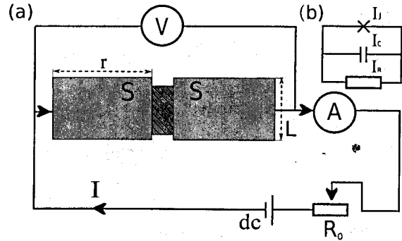
Рис. 5. (а) Джозефсоновский переход в электрической цепи [31]. Переход имеет ширину L в поперечном направлении и \tau в продольном. (б) Схематическое представление ДП в рамках RCSJ-модели. I_J , I_C и I_R токи Джозефсона, смещения и квазичастичный, соответственно.
