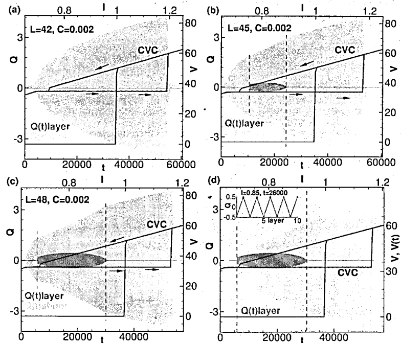
Рис. 4. Временная зависимость заряда на шунтирующем конденсаторе (светлый, голубой) и заряда в S -слоях (темный, оранжевый) вместе с соответствующей частью ВАХ, включающей rc -ветку, рассчитанную для системы десяти ДП, емкостью C = 0.002 и индуктивностью (a) L = 42 , (b) L = 45 , (c) L = 48 . (d) временная зависимость напряжения и заряда с соответствующей частью ВАХ системы N = 10 ДП, шунтированной резонансным контуром с \omega_{rc}^p = 3.2596 . Вставка показывает продольную плазменную волну с длиной волны \lambda = 2 , которая появляется в стеке при I = 0.85 .
