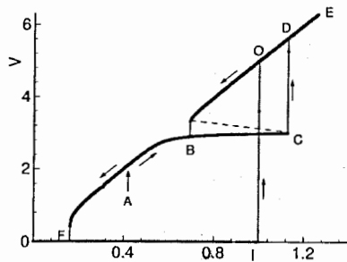
Рис. 2. ВАХ одного шунтированного ДП, рассчитанная при увеличении и уменьшении базового тока. Стрелки указывают направление изменения тока.
