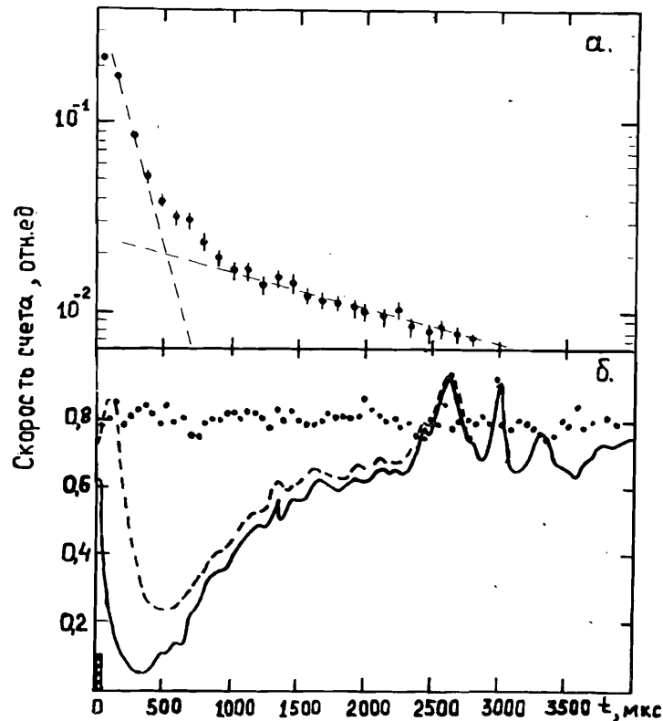
Рис. 4. Временная структура отклика канала в импульсном поле нейтронов за защитой ускорителя при L = 80 м, U = 960 В: а) в рабочем режиме при v = 240 мВ; б) в проверочном режиме при v \approx 20 мВ. Точками обозначена скорость счета шумов коронного разряда при неработающем ускорителе, сплошной линией — шумов коронного разряда при работающем ускорителе, пунктирной линией — сумма шумов коронного разряда и импульсов нейтронов при работающем ускорителе. Маркер в начале координат соответствует длительности сброса пучка ускорителя.
