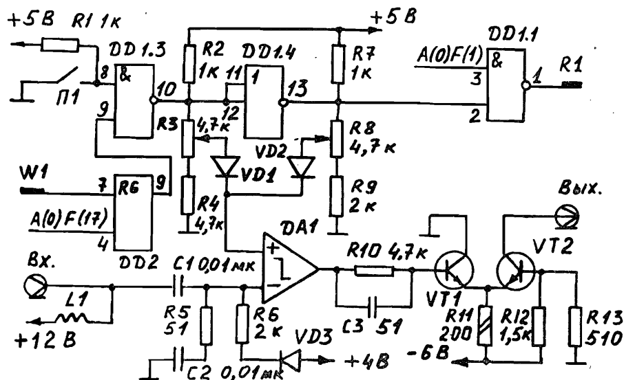
Рис. 2. Принципиальная схема дискриминатора-формирователя. DA1-K521CA2, DD1-K155ЛАЗ, DD2-K155ТМ7, VT1, VT2-KT315, VD1, VD2, VD3-Д310, L1-ДМ-0,1-400.
