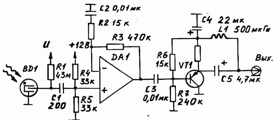
Рис. 1. Принципиальная схема усилителя датчика нейтронов. ВД1-СНМ-14, DA1-К574УД1, VT1-ГТ308.
