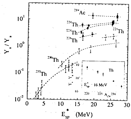
Рис.8. Y_s/Y_a в зависимости от энергии возбуждения E_{sp}^* для делящихся ядер ^{219}\text{Ac} и для цепочек Th. Данные: ^{219}\text{Ac} , ^{220,224,226}\text{Th} - настоящая работа; ^{229,230,233}\text{Th} - другие работы.
