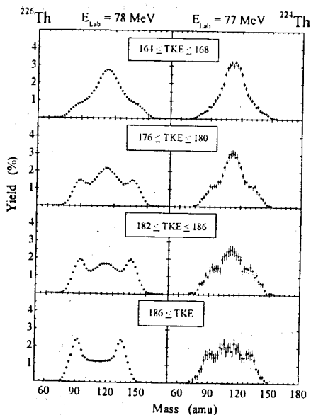
Рис.9. Изменение массовых распределений ^{224,226}\text{Th} в зависимости от полной кинетической энергии осколков ТКЕ.
