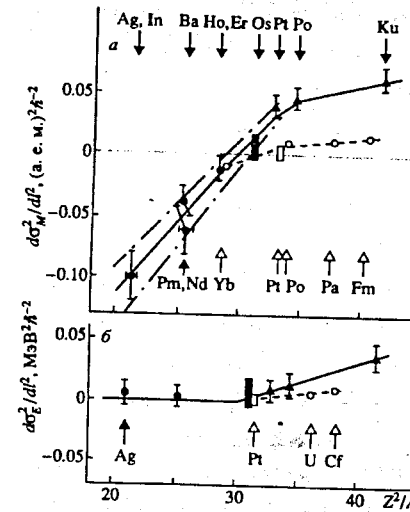
Рис.2. Коэффициенты чувствительности d\sigma_M^2/d\ell^2 (а) и d\sigma_E^2/d\ell^2 (б) в зависимости от Z^2/A . Точки: ●, ■ - результаты настоящего анализа для указанных ядер ( Ku = {}^{260}104 ), ▲ - данные других работ для \theta_{sp}^{eff} = 1.5 \text{ МэВ} ; ○ - теоретические расчеты [17]. Сплошные линии проведены по экспериментальным точкам, штриховые - по теоретическим; штрихпунктирные - коридор ошибок для оценки погрешности результатов.
