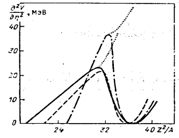
Рис.1. Зависимость жесткости ядер d^2V/d\eta^2 к масс-асимметричным деформациям от параметра делимости Z^2/A [17]: сплошная, штрихпунктирная, пунктирные кривые — МЖК [9], [7], [10] соответственно для седловой точки; пунктирная - для точки разрыва.
