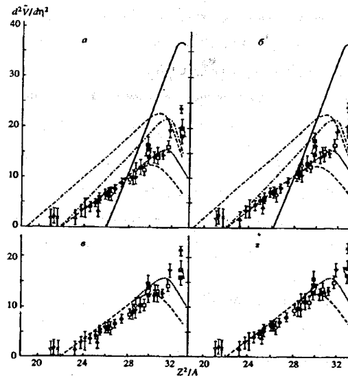
Рис.3. Зависимость жесткости d^2V/d\eta^2 от Z^2/A , вычисленной по \theta_{sp}^{eff} и \sigma_M^2 , поправленным на \ell согласно сплошной линии на рис.2. Теоретические кривые: сплошная - [6], штриховая с двумя точками - [9], штрихпунктирная - [10], штриховая - [18] с параметрами из [13]. Данные: ● - настоящая работа, остальные значки - наш анализ других работ.
