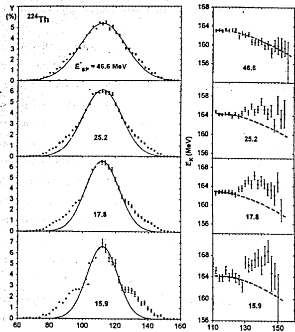
Рис.4. Выходы Y и полные кинетические энергии осколков в зависимости от массы M для деления компаунд - ядра ^{224}\text{Th} при нескольких энергиях возбуждения E_{sp}^* . Сплошные кривые - описание Y_s гауссианом, штриховые - жидкокапельная параболическая зависимость E_k(M) .
