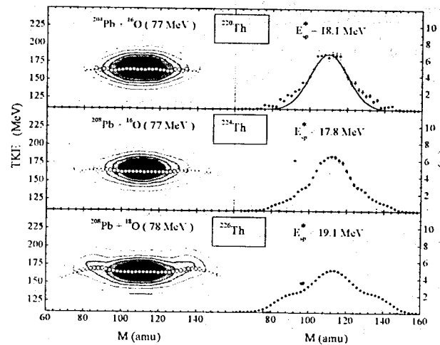
Рис.6. Слева: двумерные матрицы (полная кинетическая энергия ТКЕ*масса) осколков деления ядер ^{226,224,220}\text{Th} при приблизительно одинаковой E_{sp}^* . Открытые кружки - экспериментальная зависимость \langle E_k \rangle(M) . Слева: соответствующие матрицам выходы масс осколков. Сплошные кривые - выход симметричного деления описанный гауссом.
