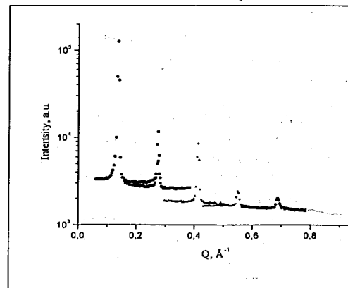
Рисунок 7. Кривые качания, измеренные при шести различных угловых положениях детектора (7, 11.2, 16.8, 22.4, 28, 33.6 градусов), для мембраны CER6/Ch/PA/ChS с соотношением компонент 55/25/15/5 (по весу). Влажность 60%, 8% D_2O , T = 32^{\circ}\text{C} .
