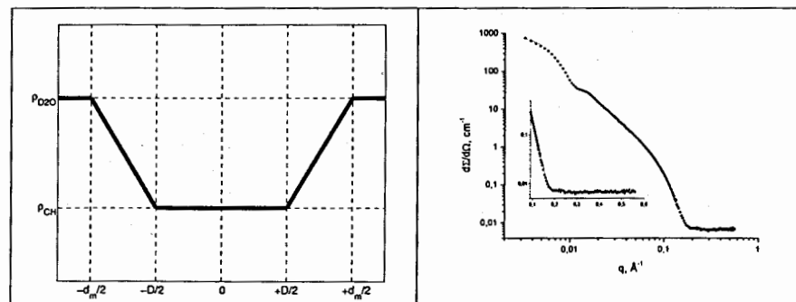
Рисунок 4. Гидрофобно-гидрофильное приближение плотности длины рассеяния нейтрона \rho(x) вдоль нормали к плоскости бислоя. Рисунок 5. Экспериментальное макроскопическое сечение рассеяния нейтронов от популяции ОСВ при T = 30^\circ C (точки) и расчетная кривая в ГГ приближении.
