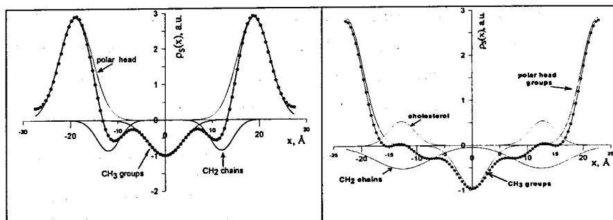
Рисунок 8. Распределение плотности длины рассеяния нейтрона \rho_s(x) в однослойной мембране ДМФХ при RH = 60\% , T = 32^\circ\text{C} и 8\% содержании \text{D}_2\text{O} (точки) и расчетные кривые (сплошная линия). Стрелки показывают положение трех молекулярных групп: \text{CH}_3 группы, \text{CH}_2 цепочки и группы полярных голов.
