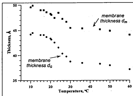
Рисунок 6. Зависимость толщины мембраны ДМФХ d_G и толщины мембраны d_m от температуры. Величина d_G определена из спектра МУРН в приближении Гинье. Величина d_m рассчитывается на основе поправок, сделанных по результатам расчетов на основе РФФ метода [10].
