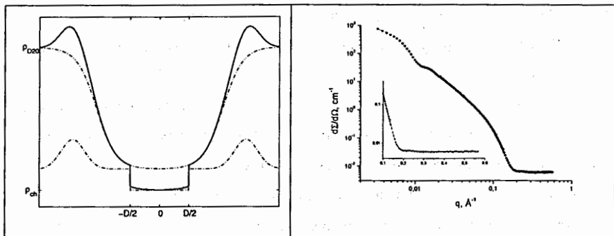
Рисунок 2. Приближение \rho(x) гауссовыми функциями. Плотность длины рассеяния «сухого» бислоя (---) линия, D_2O — (---) линия, результирующая сумма — сплошная линия. Флуктуационное приближение. Рисунок 3. Экспериментальное макроскопическое сечение рассеяния от везикул ДМФХ при T = 30^\circ C (точки) и расчетная кривая (линия) в флуктуационном приближении. На вставке показана часть спектра в области больших q .
