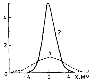
Рис. 3. Распределение интенсивности пучка атомов натрия в поперечном сечении. 1 - исходный тепловой пучок. 2 - пучок после облучения аксиально-симметричным лазерным полем на длине около 3 см.
