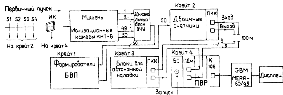
Рис.1. Блок-схема установки. S1-S4 - мониторные счетчики, ИК - ионизационная камера, ЗЧУ - зарядово-чувствительные усилители, ПКК - контроллер типа L, последовательный драйвер магистрали, К 106 - интерфейс СМ-3 типа 106А, БВП - блоки высоковольтного питания, ПВР - параллельный входной регистр, БС - блок синхронизации.
