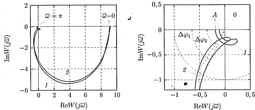
Рис. 16: Амплитудно-фазовые частотные характеристики разомкнутой системы при представлении реакторов ИБР-2 (1) и ИБР-2М (2) без автоматического регулятора в виде одноконтурной замкнутой системы при средней мощности 2 МВт. Справа более детально представлены участки характеристики вблизи нуля
