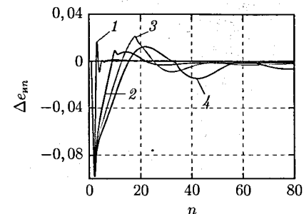
Рис. 4: Относительное отклонение энергии импульсов мощности \Delta \epsilon_{mn} при скачке реактивности (в долях \beta_n ) r_F = -0,1 ; для второго варианта АР. 1 – параметр АР N = 1 ; 2 – N = 8 ; 3 – N = 16 и 4 – N = 32 ; n – номер импульса мощности
