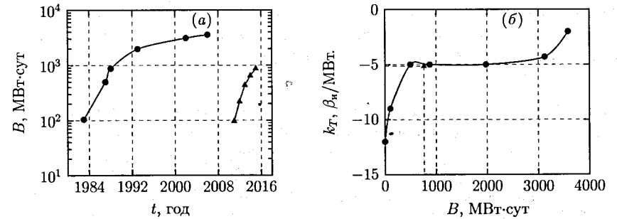
Рис. 13: Энерговыработка импульсных реакторов ИБР-2 (●) и ИБР-2М (▲) в зависимости от времени работы реактора (а) и суммарный коэффициент мощностной обратной связи ИБР-2 ( k_T ) в зависимости от энерговыработки для ИБР-2 и при энерговыработке \sim 850 МВт-сут для ИБР-2М (б)
