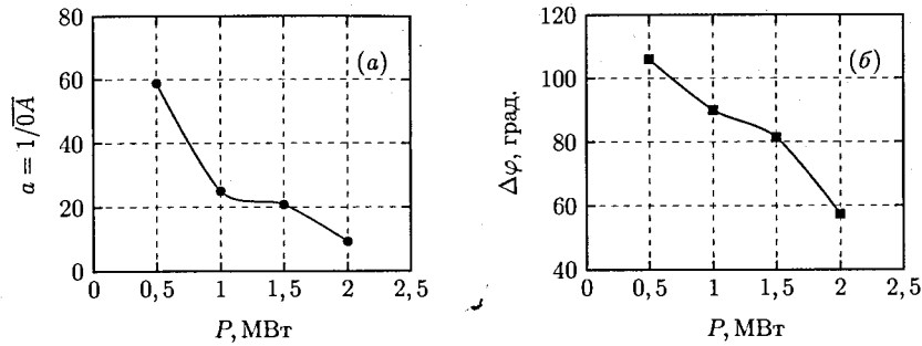
Рис. 10: Зависимости запасов устойчивости по амплитуде (а) и фазе (б) от средней мощности импульсного реактора ИБР-2М
