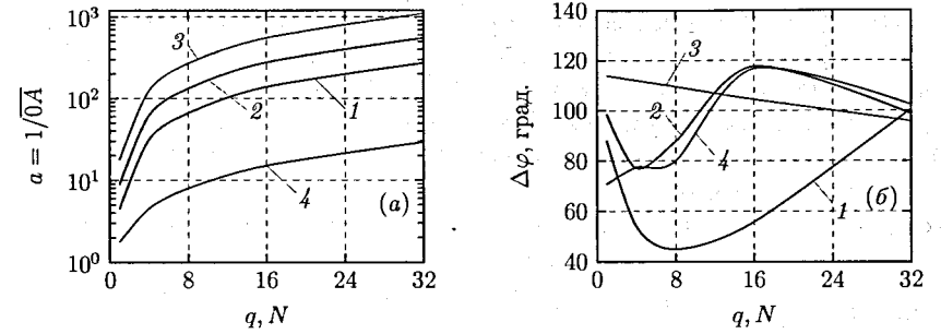
Рис. 12: Запас по амплитуде (а) и фазе (б): для первого варианта АР 1 – \Delta = 0,05 , 2 – \Delta = 0,1 и 3 – \Delta = 0,2 ; для второго варианта АР – 4
