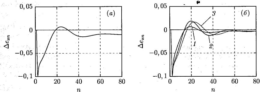
Рис. 3: Относительное отклонение энергии импульсов мощности \Delta \epsilon_{mn} при скачке реактивности (в долях \beta_n ) r_F = -0,1 для первого варианта АР. а) АР отключен (режим саморегулирования); б) АР включен, параметр фильтра q = 1 (1); 8 (2); 32 (3) при \Delta = 0,2 ; n – номер импульса мощности
