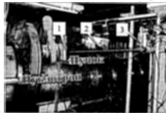
Рисунок 3 – Фотография прототипа облучательного стенда. 1 – окно вывода пучка; 2, 3 – детекторы системы мониторинга пучка.
