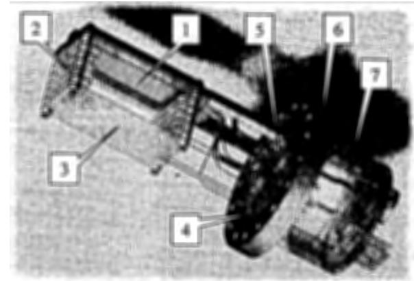
Рисунок 1 – Трехмерная модель детектора для диагностики радиальной координаты пучка Нуклотрона. 1 – запирающий электрод, шевронная сборка МКП и печатная плата с многоканальным коллатором; 2 – электроды, выравнивающие электростатическое поле транспортировки ионов; 3 – ускоряющий электрод; 4 – высоковольтные вакуумные разъемы; 5 – сигнальные вакуумные разъемы; 6 – вакуумный фланец; 7 – короб для защиты вакуумных разъемов.
