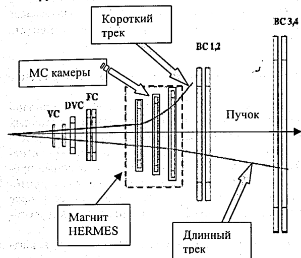
Рис. 16. Трековая система. Принцип разделения длинных и коротких треков.
