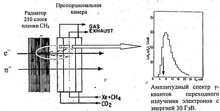
Рис.2. Модуль ДПИ
