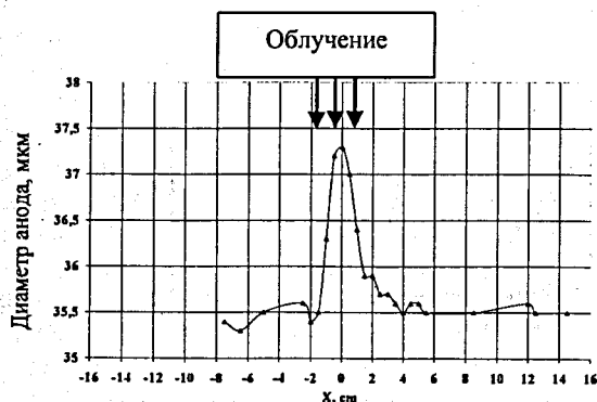
Рис.20а. Эффект распухания анодной проволочки. Зависимость диаметра проволочки от координаты вдоль проволочки.
