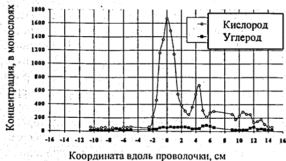
Рис.20б. Распределения концентрации кислорода и углерода вдоль проволочки, полученные методом NRA.
