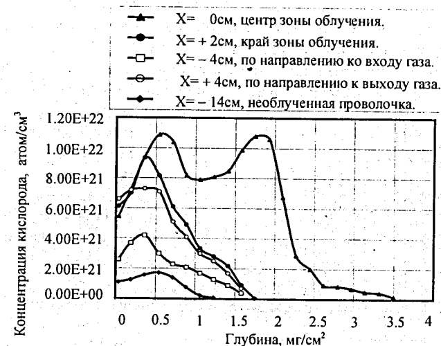
Рис.19. Распределение концентрации кислорода как функция глубины золотого покрытия в различных точках вдоль анодной проволоочки. Ориентировочный масштаб: 1 \text{ мг/см}^2 соответствует 0,5мкм по толщине.
