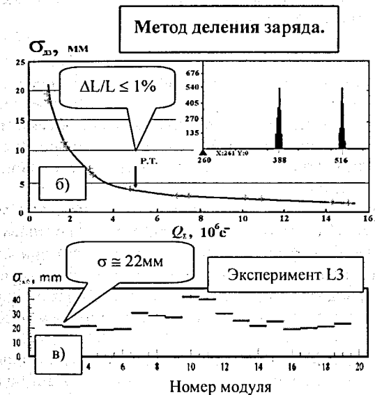
Рис. 15. Пространственное разрешение FTC.
