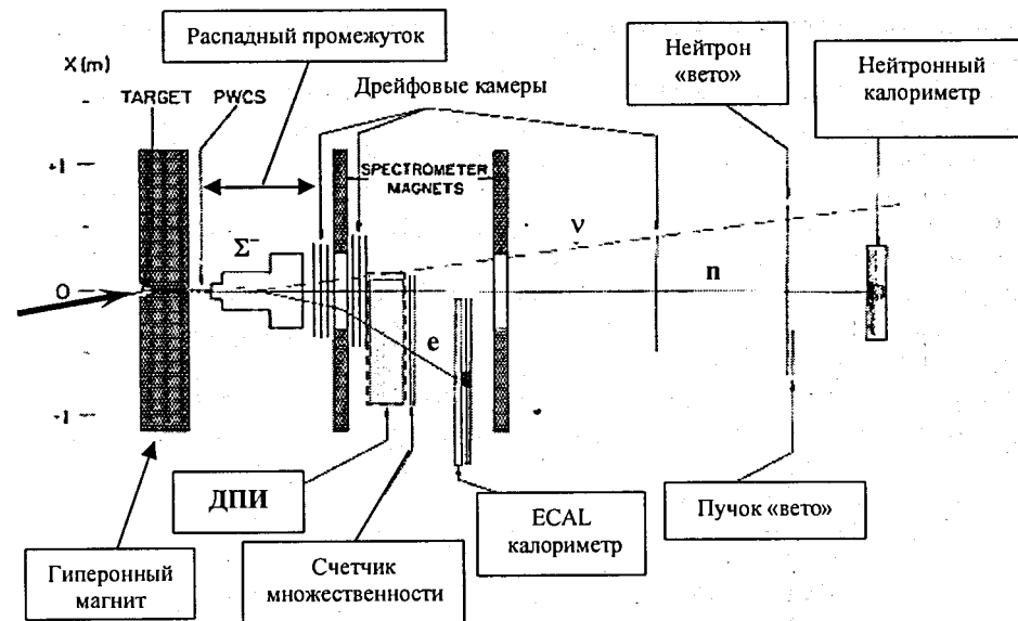
Рис.1. Экспериментальная установка по исследованию \beta распада \Sigma^- гиперонов.
