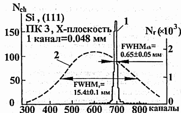
Рис.12. Пространственное расположение пучка на X плоскости (ПКЗ): 1 — с отбором по критерию малой амплитуды сигнала с детектора (в интервале 0.3±0.6 от наиболее вероятного значения для хаотической фазы), 2 — без отбора (прямой пучок).
