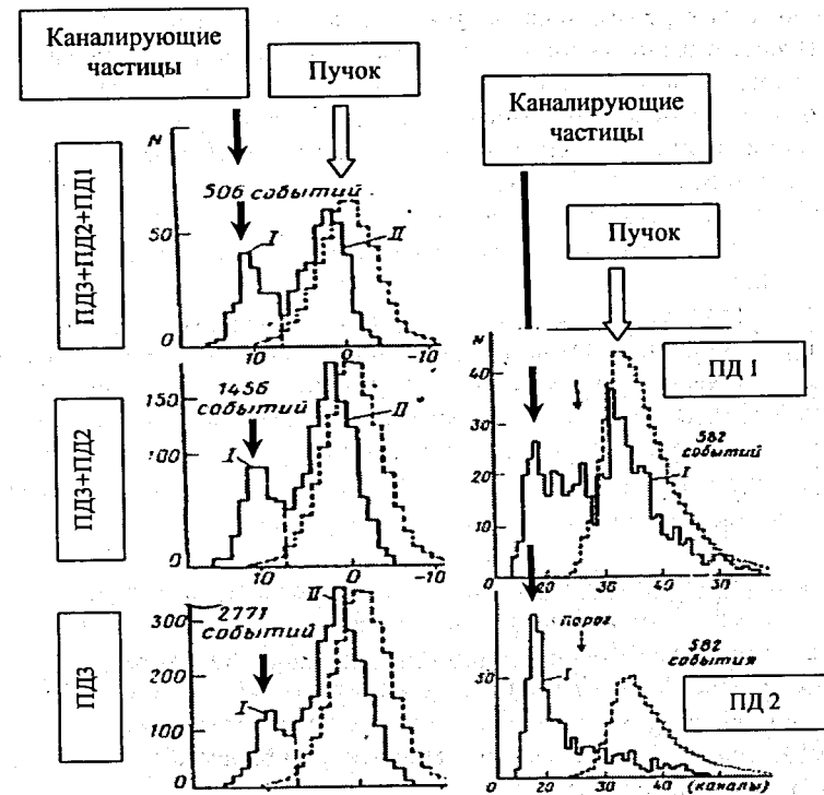
Рис.11а. Угловые распределения частиц, прошедших кристалл с отбором по критерию малой амплитуды. Угол поворота \phi = 11 мрад.
