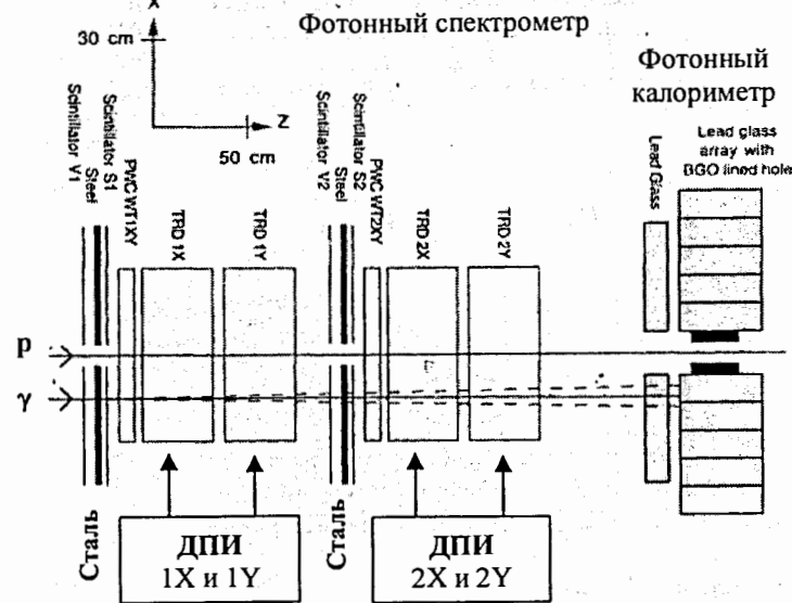
Рис.7. Фотонный спектрометр. Положение электромагнитного ливня в стальном конверторе измеряется пропорциональными камерами (PWC) и ДПИ (TRD). Энергия фотонов измеряется в фотонном калориметре.
