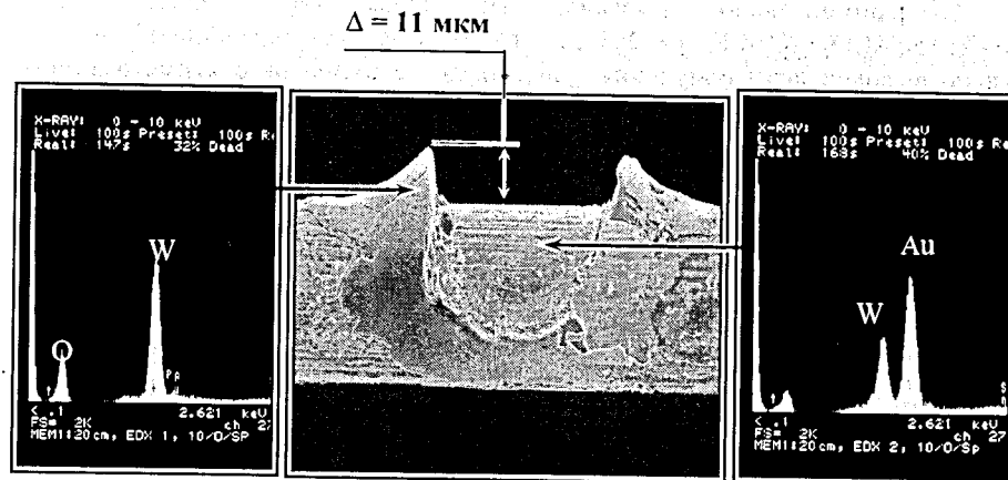
Рис.21. Типичные результаты обследования анодной проволочки методом SEM/XEM в точке, расположенной вблизи зоны облучения со стороны выхода газового потока. Очень толстый слой (11мкм) окиси вольфрама хорошо наблюдается поверх золотого покрытия проволочки. Диаметр проволочки – 30мкм.
