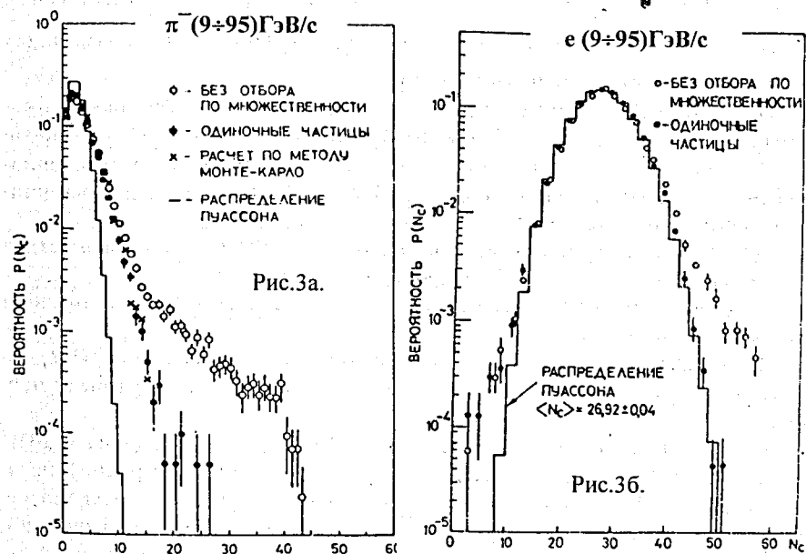
Рис.3. Распределение по числу зарегистрированных кластеров для \pi^- -мезонов (Рис.3а) и для электронов (Рис.3б). Значение параметра \lambda , используемое для построения распределения Пуассона, получено из соотношения \lambda = -\ln P(0) , где P(0) - вероятность не зарегистрировать ни одного кластера на одну прошедшую частицу.
