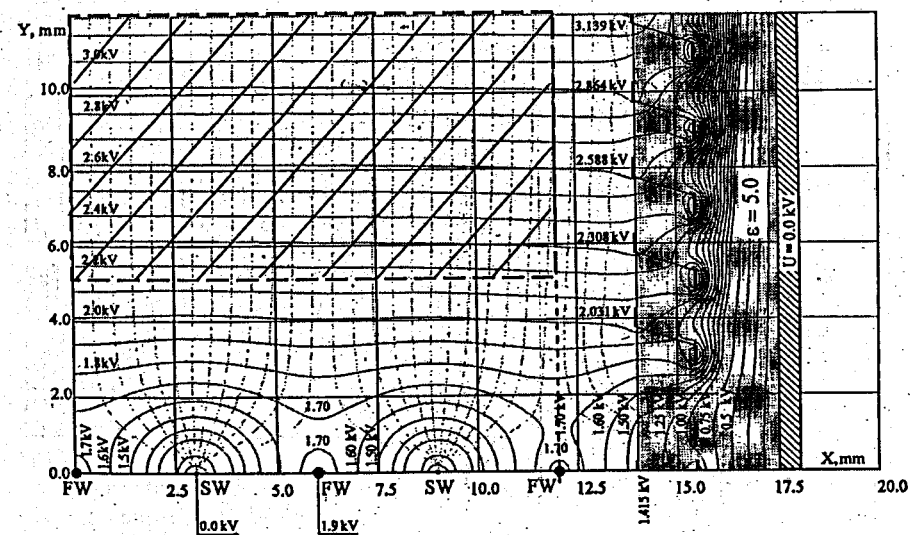
Рис.14. Компьютерная симуляция структуры электрического поля в модуле FTC при наличии двух слоёв полеформирующих стрипови заземлённого защитного экрана, установленного в 3,5 мм от границы внутреннего объёма. Внешний слой стрипов смещён на 1мм вниз относительно внутреннего.
