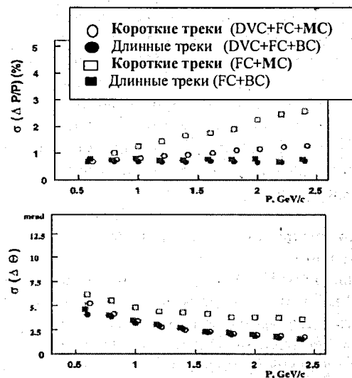
Рис. 17. Импульсное и угловое разрешения, полученные для коротких и длинных треков, при различных комбинациях использования информации с различных трековых детекторов.
