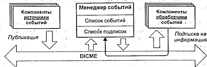
Рис. 4. Схема работы менеджера событий и компонента DiCME при обслуживании вспомогательных операций
