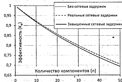
Рис. 8. Оценка влияния использования компонента DiCME на эффективность работы САЭ
