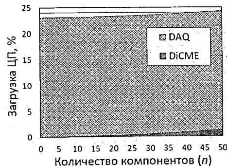
Рис. 5. Влияние использования компонента DiCME на загрузку ЦП
