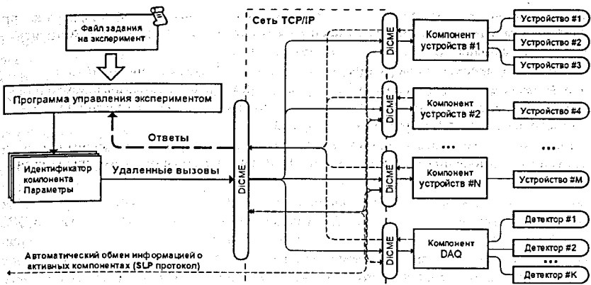
Рис. 3. Схема взаимодействия программы управления экспериментом и компонента DiCME при реализации основных задач ПО САЭ
