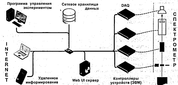
Рис. 1. Пример схемы распределенной САЭ
