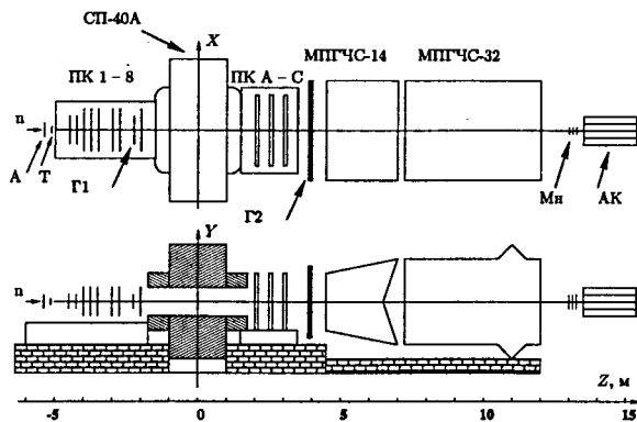
Рис. 1: Спектрометр ЭКСЧАРМ.
