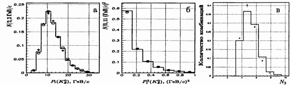
Рис. 3: (а), (б) импульсные спектры K_S^0 -мезонов; (в) — распределение по множественности заряженных частиц. Здесь и на рис. 7 гистограмма — эксперимент; * — модель FRITIOF; о — перемешивание.
