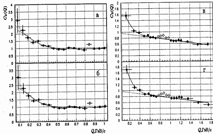
Рис. 4: Корреляционные функции C_2(Q) : (а)-(б) — для K_S^0 K_S^0 ; (в)-(г) — для K_S^0 K_S^- . ОР: (а), (в) — моделирование; (б), (г) — „двойное отношение“.
