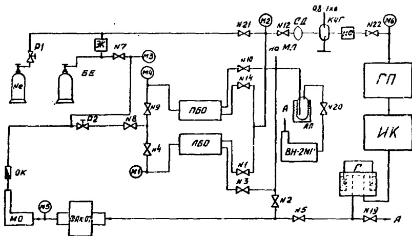
Рис. 5. Схема газообеспечения искровых камер. СД - стабилизатор давления; КЧГ - индикатор контроля чистоты газа; Г - газгольдер; ЛБО, ЛБО - правый и левый блоки очистки; АЛ - азотная ловушка; ВН-2МГ - вакуумный насос; ФАК-0,7 - компрессор; N1 - N22 - вакуумные насосы; ФАК-0,7 - компрессор; N1 - N22 - сильфонные вентили; M1-4 - мановакуумметры; M5, M6 - манометры; МО - маслоочиститель; ОК - обратный клапан; МФ - масляный фильтр; БЕ - балластная емкость; ЭК - электроклапан; А - атмосфера; МЛ - манометрическая лампа.
