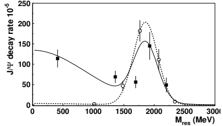
Рис. 5 — Парциальная ширина рождения изоскалярных скалярных мезонов для преимущественно синглетных (треугольники) и преимущественно октетных (квадраты) состояний [A3].
