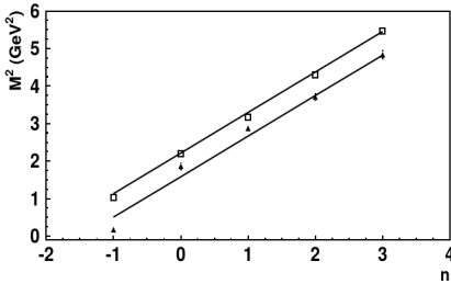
Рис. 4 — Реджеподобные линейные траектории в плоскости (n, M^2) для состояний с доминирующей синглетной (треугольники) и октетной (квадраты) компонентами флейворной волновой функции [A3].
