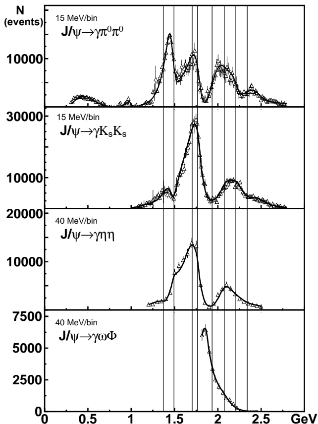
Рис. 3 — Интенсивности S -волны двух мезонов в радиационных распадах J/\psi как функции их инвариантной массы [A3]. Гистограммы а) и б) соответствуют статистике в 1,3 миллиарда распадов J/\psi , гистограммы с) и d) — статистике в 225 миллионов распадов J/\psi . Вертикальные полосы обозначают массы резонансов, полученные в аппроксимации.
