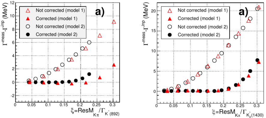
Рис. 1 — Эффективность применения метода учета разрешения детектора при определении ширины K^*(892)^\pm и K_2^*(1430)^\pm как функция \xi — отношения разрешения по инвариантной массе K^\pm\pi^0 к ширине резонанса [A1].
