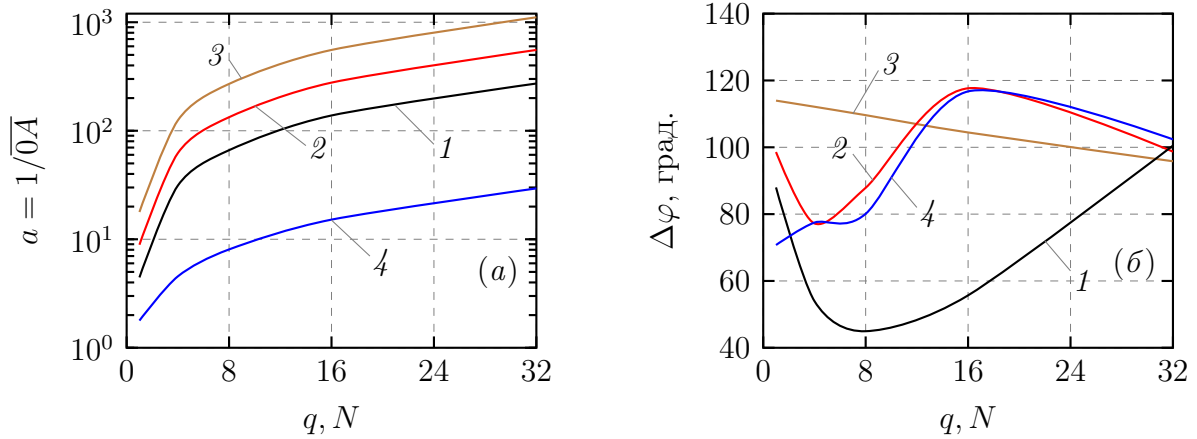
Рис. 12: Запас по амплитуде (а) и фазе (б): для первого варианта AP 1 – \Delta = 0,05 , 2 – \Delta = 0,1 и 3 – \Delta = 0,2 ; для второго варианта AP – 4
