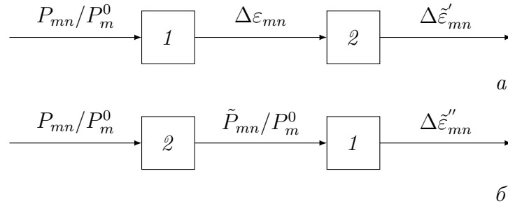
Рис. 7: Два варианта расположения статистически оптимального фильтра для получения сглаженной реактивности. 1 – реактиметер; 2 – фильтр расположения фильтра.
