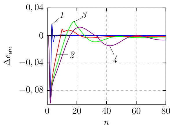
Рис. 4: Относительное отклонение энергии импульсов мощности \Delta e_{mn} при скачке реактивности (в долях \beta_n ) r_F = -0,1 ; для второго варианта АР. 1 – параметр АР N = 1 ; 2 – N = 8 ; 3 – N = 16 и 4 – N = 32 ; n – номер импульса мощности
