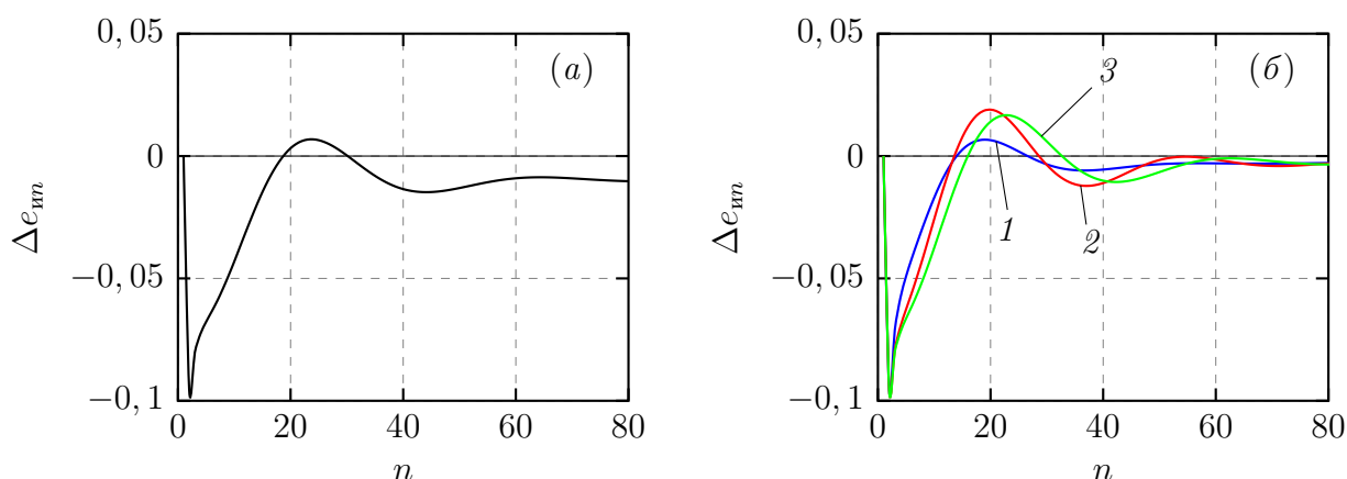
Рис. 3: Относительное отклонение энергии импульсов мощности \Delta e_{ин} при скачке реактивности (в долях \beta_{и} ) r_F = -0,1 для первого варианта АР. а) АР отключен (режим саморегулирования); б) АР включен, параметр фильтра q = 1 (1); 8 (2); 32 (3) при \Delta = 0,2 ; n – номер импульса мощности
