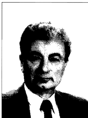
Ю.Ц.Оганесян
