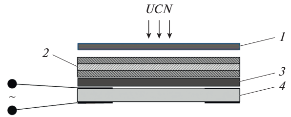
Рис. 6. Схема эксперимента: 1 – монохроматор, 2 – нейтронный интерференционный фильтр, 3 – конвертирующий слой, 4 – пьезодрайвер.
