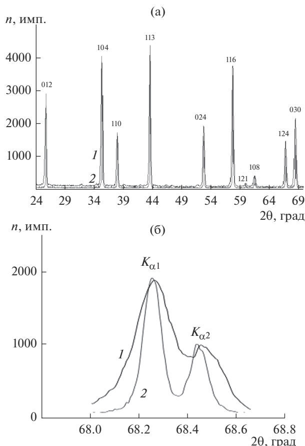
Рис. 8. Диффрактограммы Al_2O_3 , полученные на диффрактометрах: ДР-02 “РАДИАН” (1) с детектором ППД-К-12Б; X’PERT PRO PANALYTICAL (2) с детектором X’CELERATOR. Рефлексы от 012 до 030 (а). Рефлекс 030 в увеличенном масштабе (б).
