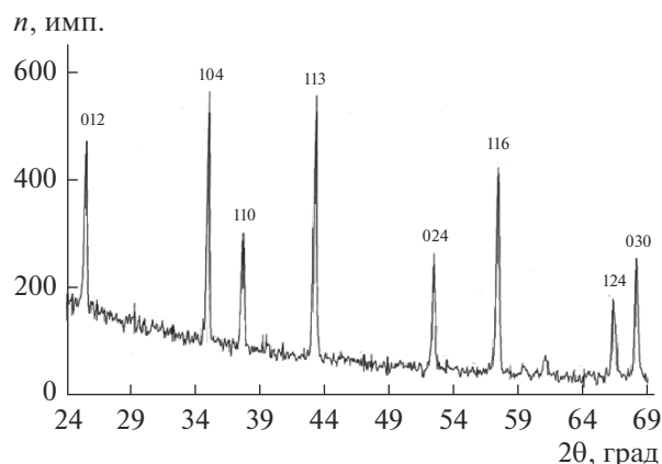
Рис. 3. Дифрактограмма \text{Al}_2\text{O}_3 , полученная с использованием сцинтилляционного детектора CsI(Tl) и никелевого \beta -фильтра толщиной 30 мкм. Здесь и далее n — количество отсчетов детектора за 1 с.
