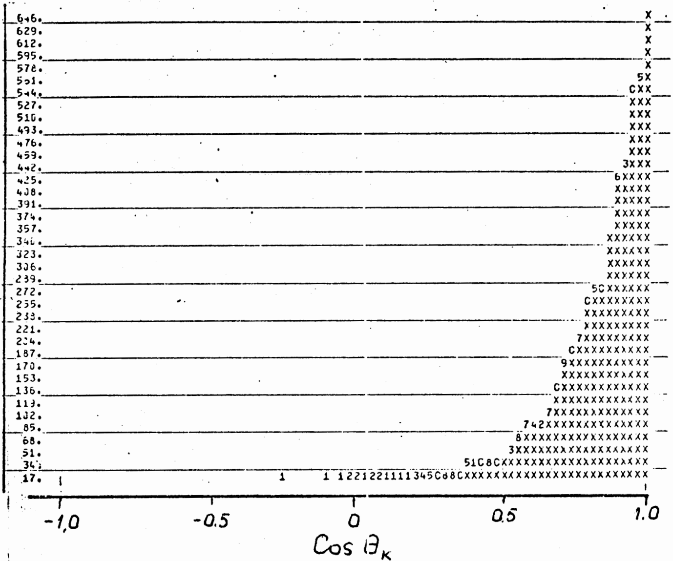
Рис.6. Угловое распределение K^+ -мезонов, рожденных совместно с релятивистскими гиперядрами {}_{\Lambda}^{16}O (результат моделирования).
