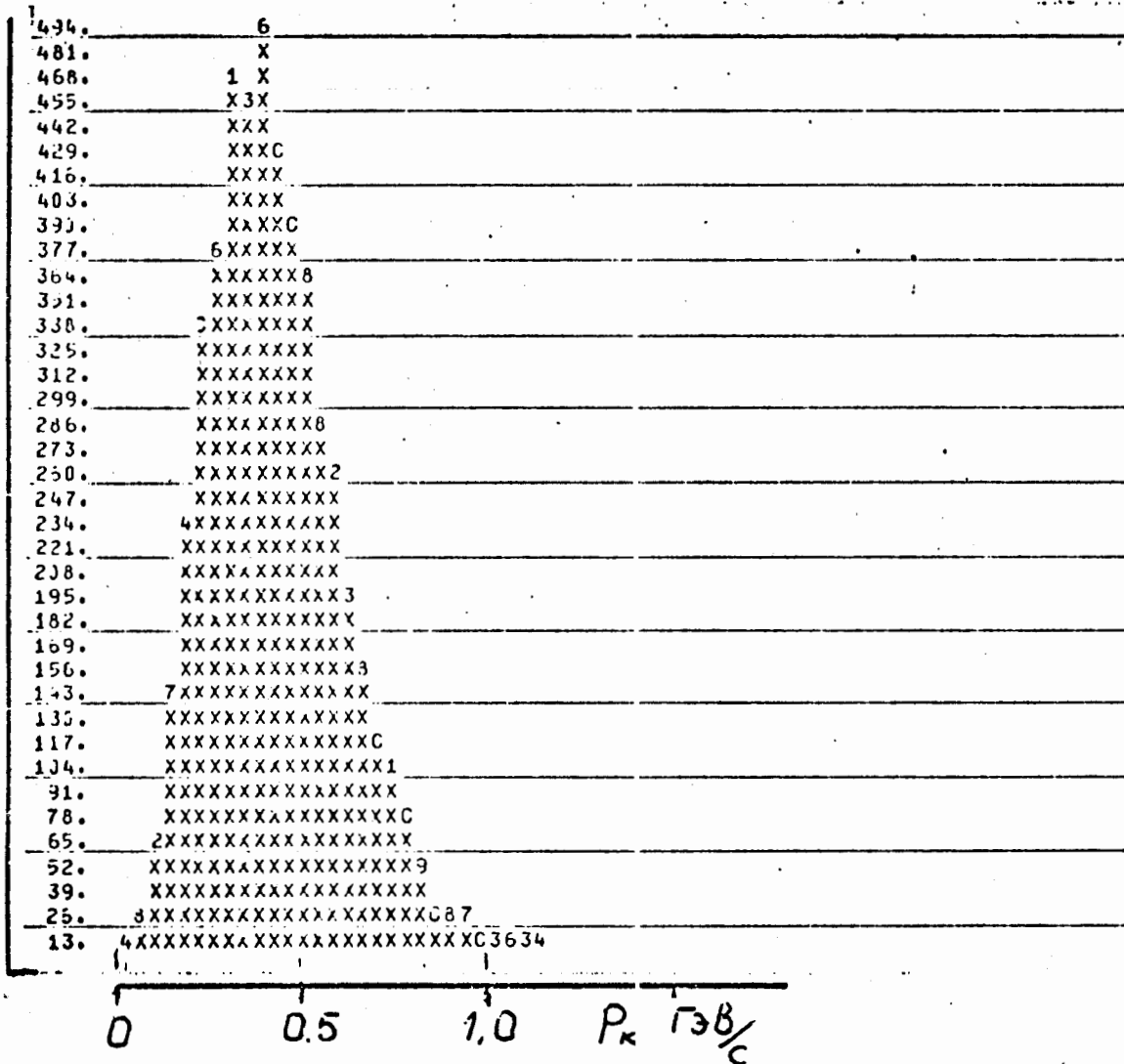
Рис.5. Импульсное распределение K + - мезонов, рожденных совместно с релятивистскими гиперядрами {}^{16}_0\Lambda (результат моделирования).
