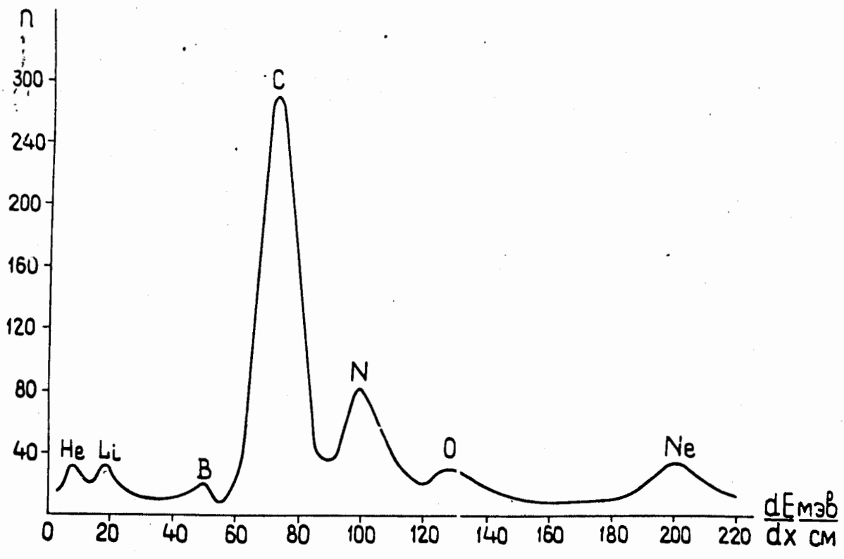
Рис.4. Амплитудное распределение ( \frac{dE}{dx} ), полученное с помощью триггерной системы установки СКМ-200, при наличии в канале смеси ускоренных ядер.
