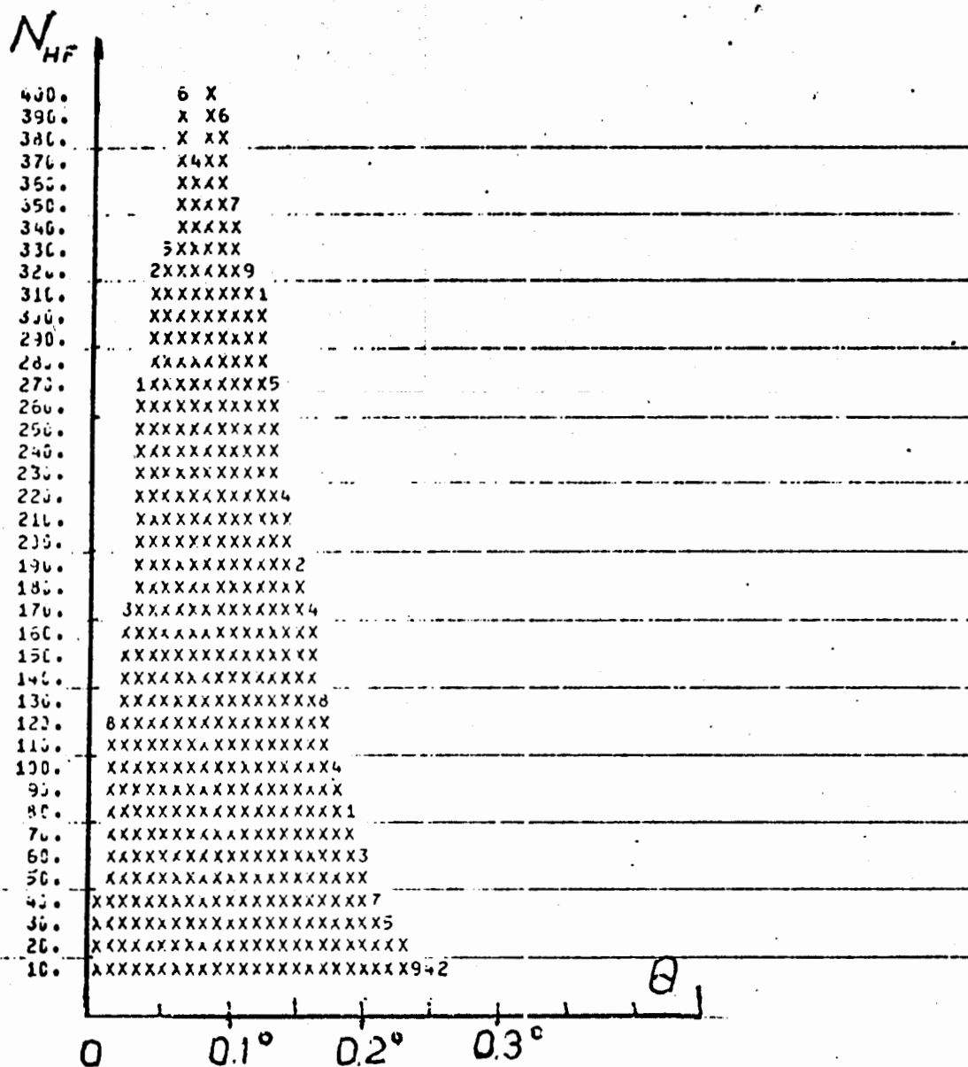
Рис.7. Угловое распределение релятивистских гиперядер {}^{16}_\Lambda\text{O} , полученных в реакции {}^{60}\text{Ni} + p \rightarrow {}^{16}_\Lambda\text{O} + K^+ + n (результат моделирования).
