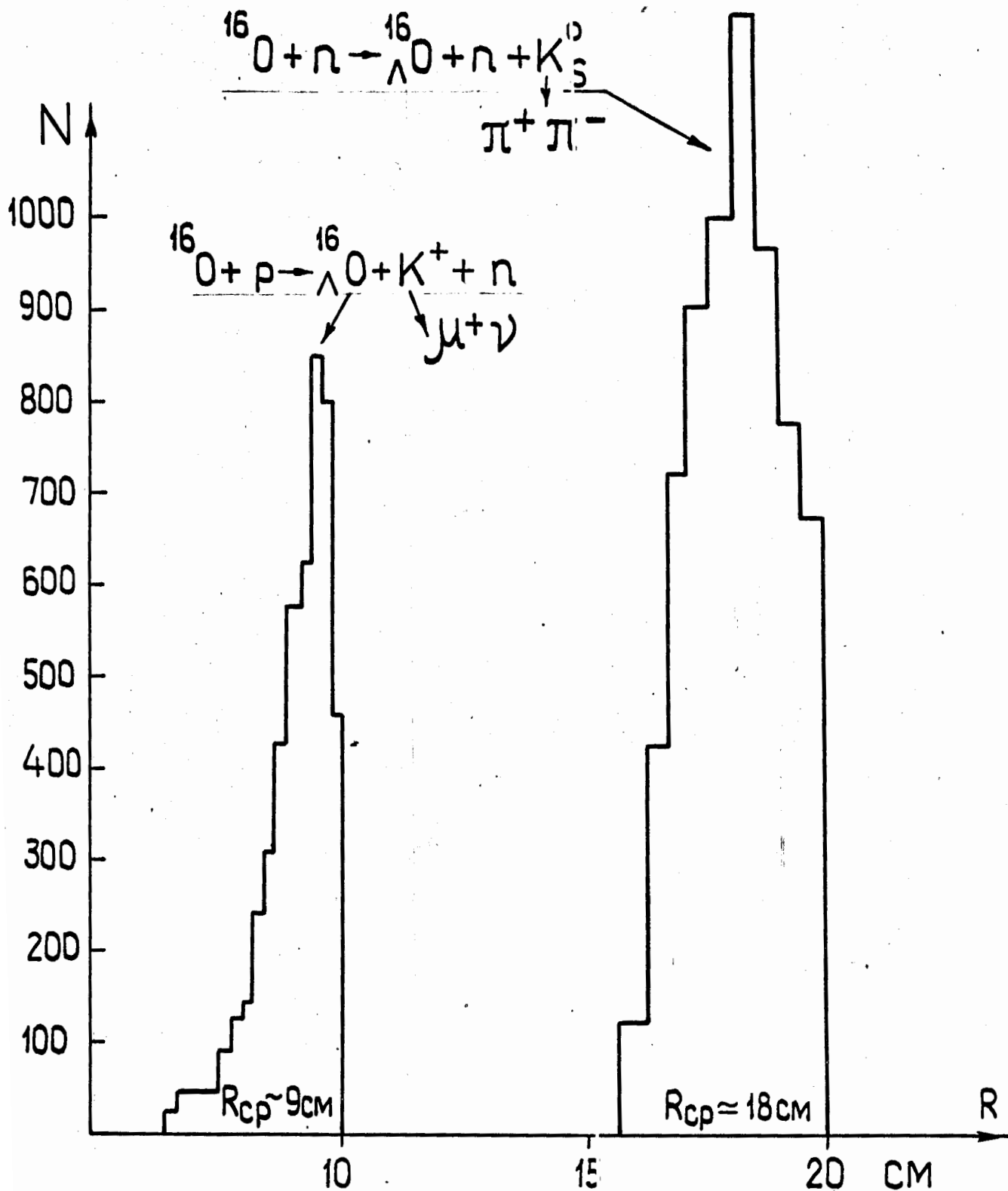
Рис. I. Распределение средних пробегов гиперядер \Lambda^{16}\text{O} полученных в соответствующих реакциях при максимальных энергиях бэвалака и синхрофазотрона при \tau = (0.86^{+0.33}_{-0.26}) \cdot 10^{-10} сек (результаты моделирования).
