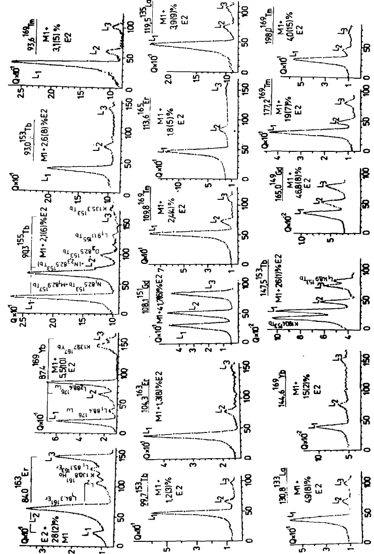
Рис.3. Фрагменты спектров, содержащие L-группы ЭК переходов смешанных M1+E2 мультипольностей. Диапазон энергий 84 < Eγ < 200 кэВ.
