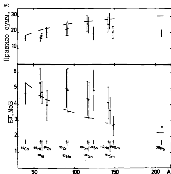
Р и с. I. Энергии центров низколежащих 3^- -возбуждений (внизу) и процент исчерпывания ЭВПС (вверху) для ядер с массовыми числами 40 \leq A \leq 210 . Расчеты для различных элементов представлены отрезками сплошных линий. Экспериментальные данные взяты из работ /21-23/ .
