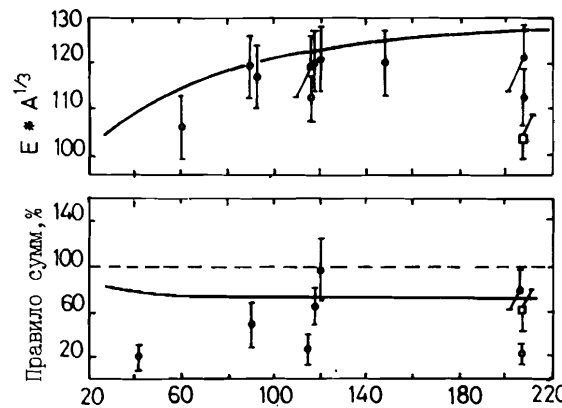
Р и с. 2. Энергии центроидов ГОР, умноженные на A^{1/3} , (вверху) и процент исчерпывания ЭВПС (внизу) для ядер с дорожки \beta -стабильности (сплошные кривые). Экспериментальные данные взяты из работы /22/ .
