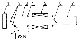
Рис.1. Схема установки для поляризационного анализа УХН в накопительном варианте с одной ловушкой: 1 - детектор УХН, 2 - заслонка, 3 - зеркальный нейтронвод, 4 - ферромагнитная пленка, 5 - спин-флиппер, 6 - заслонка, 7 - ловушка УХН.
