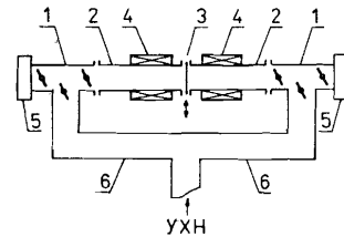
Рис.2. Схема установки для поляризационного анализа УХН в накопительном варианте с двумя ловушками: 1 - ловушка, 2 - нейтронвод, 3 - ферромагнитная пленка, 4 - спин-флиппер, 5 - детектор УХН, 6 - подводный нейтронвод.
