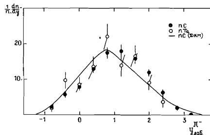
Рис.7. Распределения \pi^- - мезонов из nC - и nTa - взаимодействий по быстроте.
