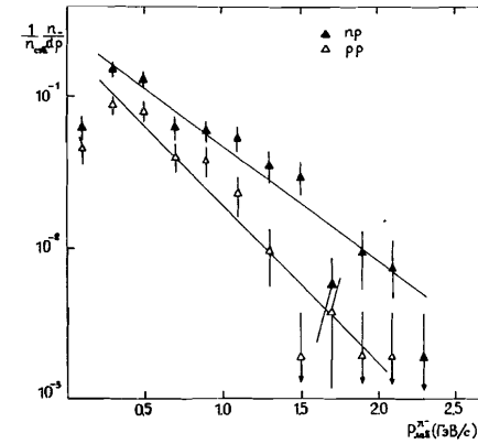
Рис. I. Импульсные спектры \Pi^- -мезонов из n p - и pp -взаимодействий. Прямые линии - результат аппроксимации спектров экспонентой.
