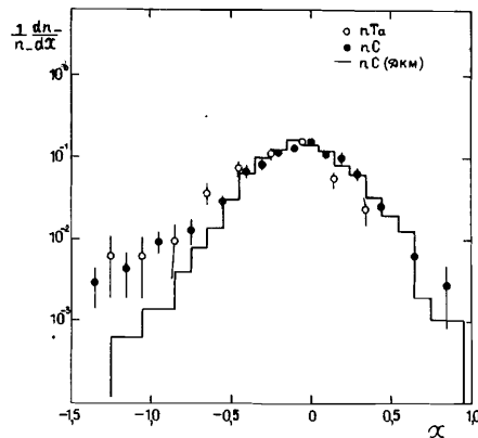
Рис.8. Распределения \pi^- - мезонов из nC^- - и nTa^- -взаимодействий по фейнмановской переменной x в системе центра масс нуклон-нуклон.
