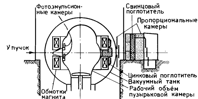
Рис. 1. Схема расположения контейнеров с фотоэмульсией внутри 15-футовой пузырьковой камеры ФНАЛ.
