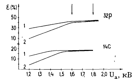
Рис. 5. Эффективность регистрации ^{32}\text{P} и ^{14}\text{C} при двух фиксированных напряжениях на промежутке предварительного усиления 8,1 кВ (1) и 8,2 кВ (2).
