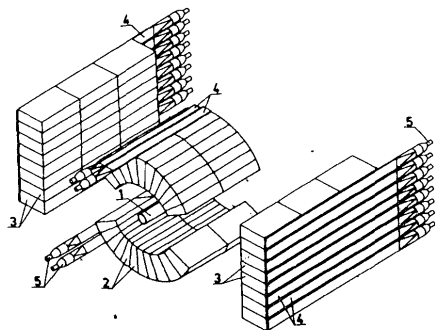
Рис.1. Схематический вид спектрометров. 1 - жидководородная мишень, 2 - блоки сцинтилляторов цилиндрического спектрометра, 3 - блоки сцинтилляторов прямоугольных спектрометров, 4 - световоды - сместители спектра, 5 - фотоумножители.
