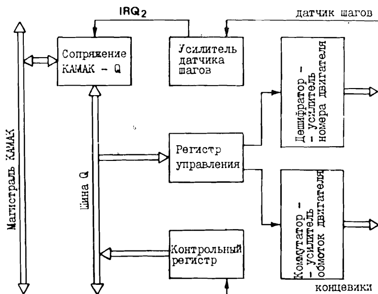
Рис. Блок-схема БУЩД-3.
