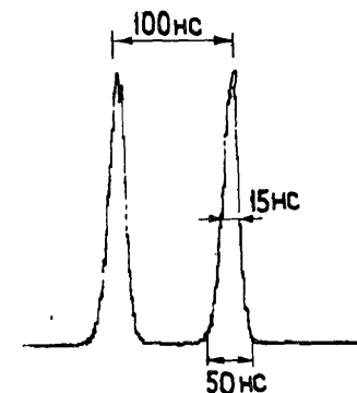
Рис. 8 Временное разрешение МСЛК для смеси Ne + 2,2\% метана.
