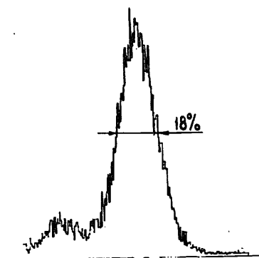
Рис.5 Типичное энергетическое разрешение МСЛК для источника ^{55}\text{Fe} .
