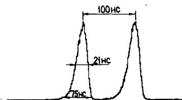
Рис.3 Типичное временное разрешение МСЛК для смеси Ar +4% ацетона.
