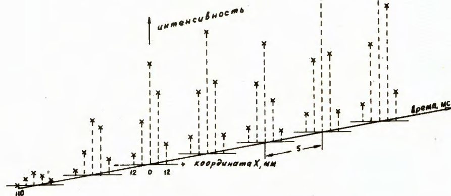
Рис.9. Изменение интенсивности во времени пучка протонов синхрофазотрона ОИЯИ в канале вывода.
