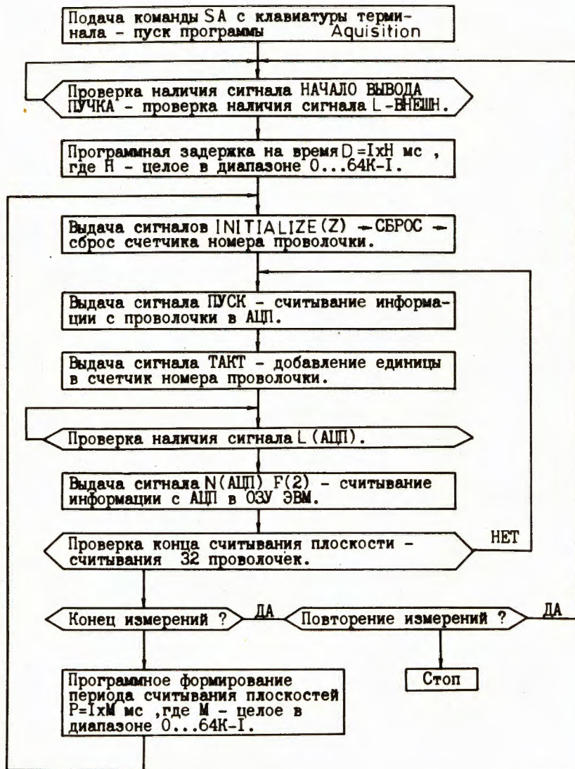
Рис.3. Организация функционирования системы диагностики.
