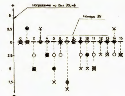
Рис.6. Выходное напряжение электрометрических усилителей с защитой на входе в виде коллекторного перехода транзистора КТ326 в зависимости от температуры и входных условий. ■ - при температуре 20°C, R_{вх} = 5,6 \text{ МОм} /обеспечивалось подстройкой нуля операционного усилителя/; o - при температуре 20°C, R_{вх} = 0 . При температуре 40°C: ● - R_{вх} = 5,6 \text{ МОм} ; x - R_{вх} = 0 .
