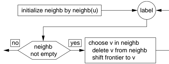
Fig. 3.10 SHIFTFRONTIERTONEIGHB( u )
