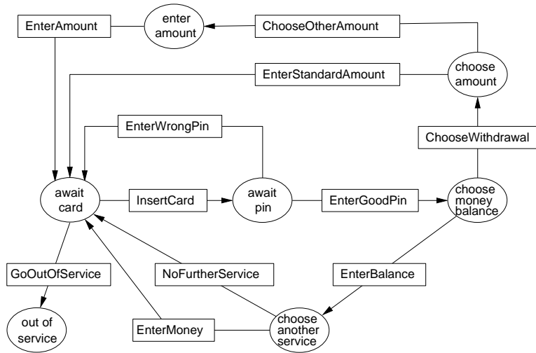
Fig. 3.2 REFINEDATM use case model
